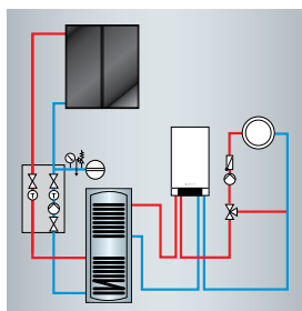
Przykładowy system grzewczy z kotłem Vitodens 200-W i kolektorami Vitosol do podgrzewu c.w.u.
