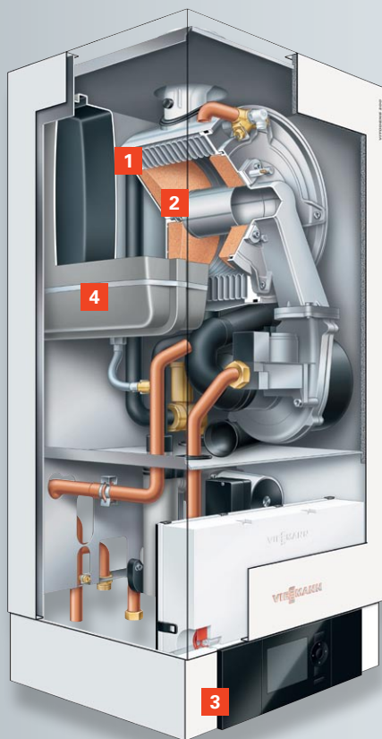
Vitodens 200-W
